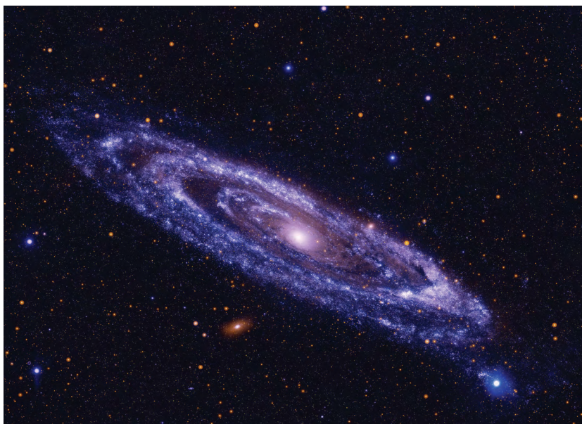
仙女座星系是安拉创造的数十亿个星系之一。它由波斯天文学家 阿布都拉合曼艾-苏菲发现于公元964年
