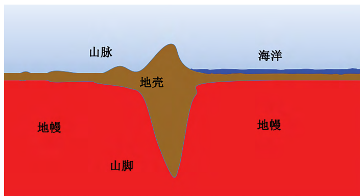
插图显示山脚深入地幔。
